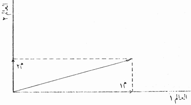
شكل ٩: تراكب العوالم:
