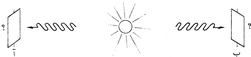
شكل ١٧: أحجية آينشتاين-روزن-بودولسكي:
