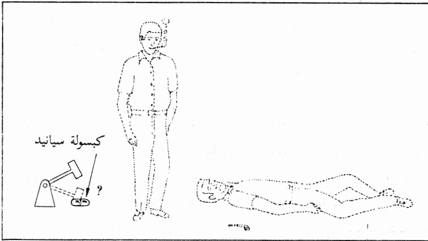
شكل ١٨: مفارقة صديق ويعثر:
