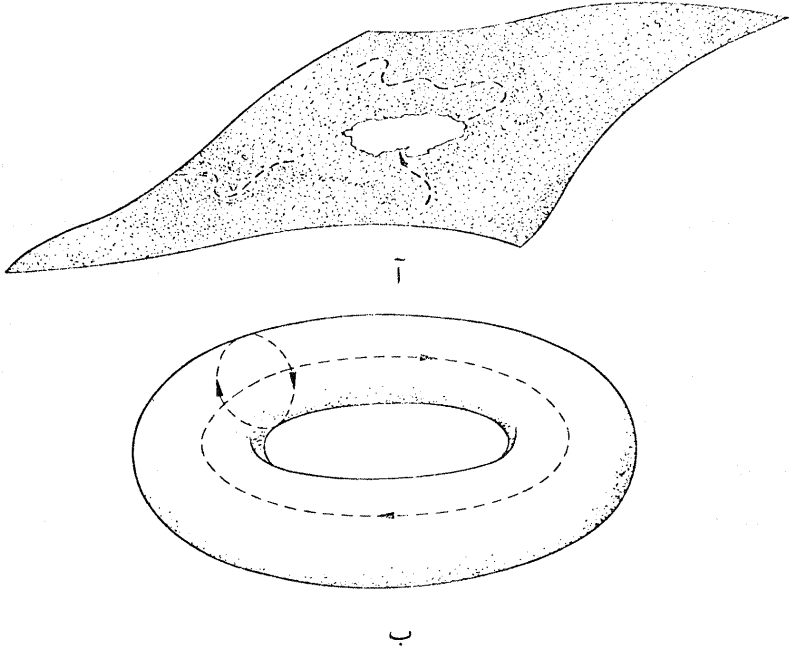
شكل ١٠: ثقوب في الفضاء:
