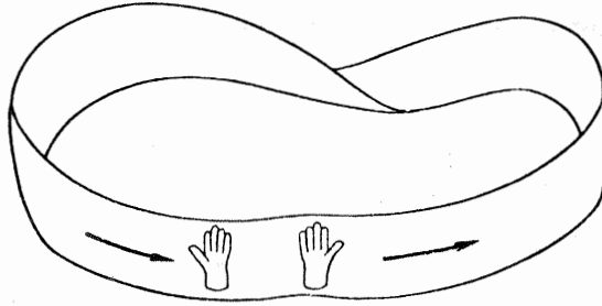
شكل ١٢: عصاة مويوس:
