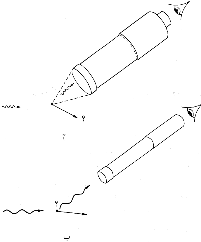
شكل ٧: مبدأ الانزياح:
