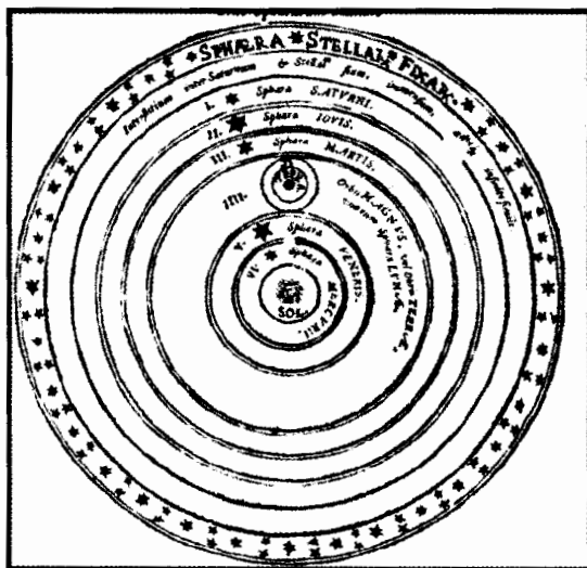
4 - نسخة قديمة تصور الشمس مركزا للكون من
