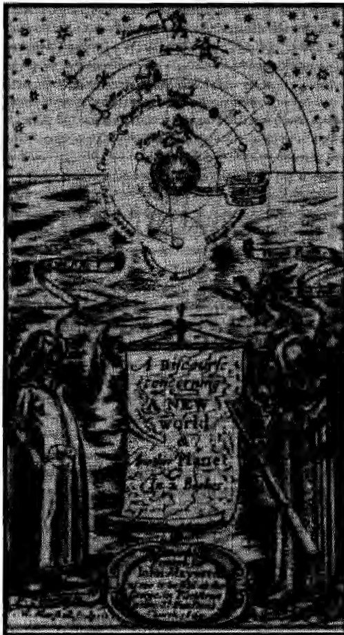
9 - كوبرنيكس وكبلر وغاليليو مع تلسكوبه والنموذج الجديد للكون مأخوذ من معرض إنجليزي قديم لهذه الأفكار، 1640.
