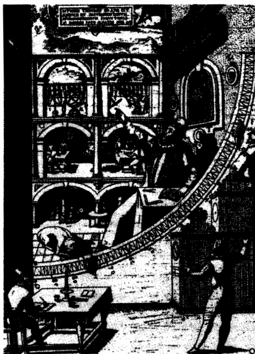
7 - تيشو والريمية الكبرى، 1569
