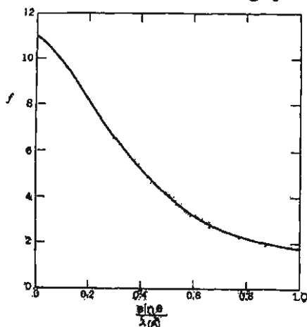
شكل (2.8): عامل التشتت الذري للصوديوم.
