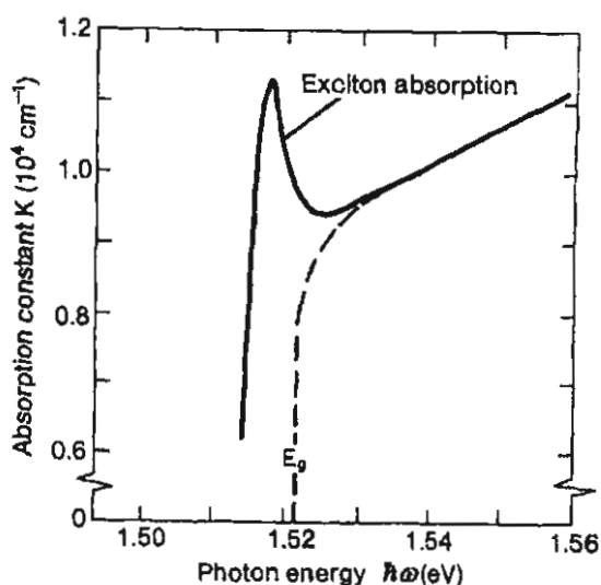
الشكل (7.9): قياس معامل الامتصاص عند درجة حرارة 21K لمادة GaAs بالقرب من الفجوة الطاقية حيث يظهر خط امتصاص الاكستون.
