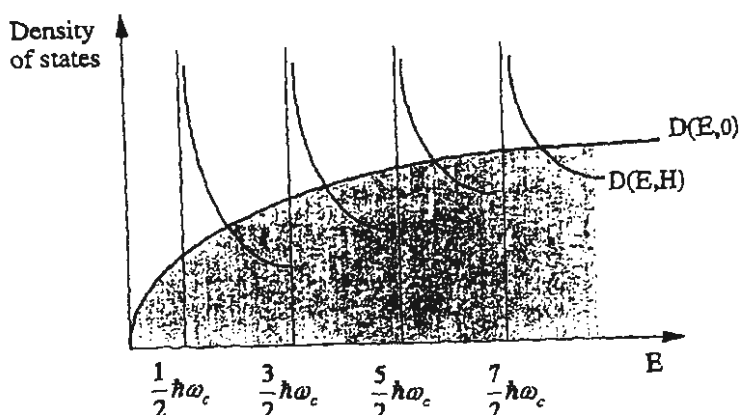
شكل (6.21): كثافة الحالات للفاز الإلكتروني عند وجوده
