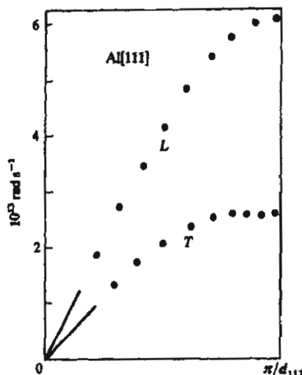
الشكل (3.7): طيف الأنماط الاهتزازية للألمنيوم في الاتجاه [111].
