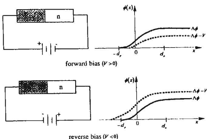
الشكل (10.16): الوصل المباشر، والوصل المعاكس للمفصل p-n.
