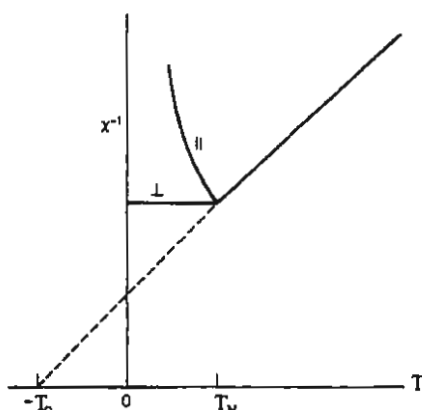
الشكل (8.15): اعتماد مقلوب القابلية المغناطيسية على درجة الحرارة لمادة فرومغناطيسية - ضدية.
