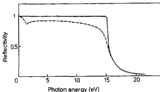
الشكل (7.5): معامل الانعكاس للفلز الحر
