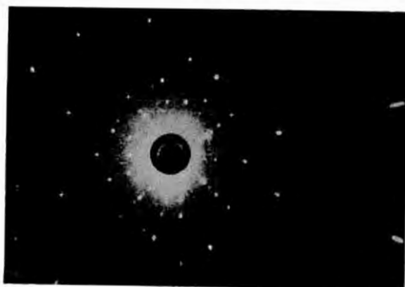
شكل (2.11): نموذج لافو لبلورة السيليكون.
