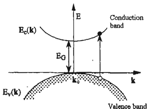
الشكل (7.6): تمثيل الانتقالات المباشرة
