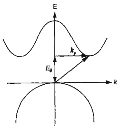
الشكل (7.10): الانتقالات غير المباشرة وفيه يظهر المتجه الموجي للفونون.
