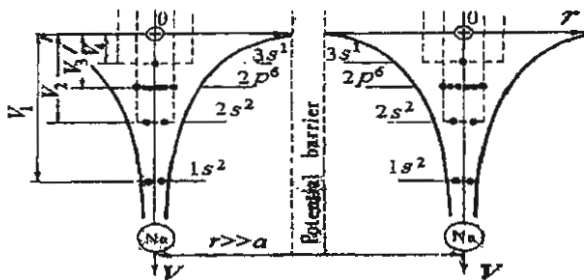
شكل (6.9): مستويات الطاقة لذرات الصوديوم عندما تكون بعيدة عن بعضها البعض ( r \gg a ).
