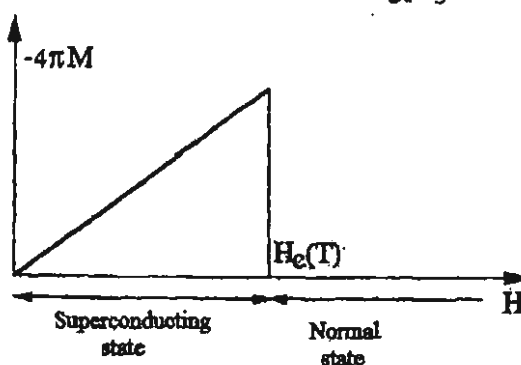
الشكل (9.4): تغير شدة التماغنط مع المجال المغناطيسي للنوع الأول I من المواد فائقة التوصيل.
