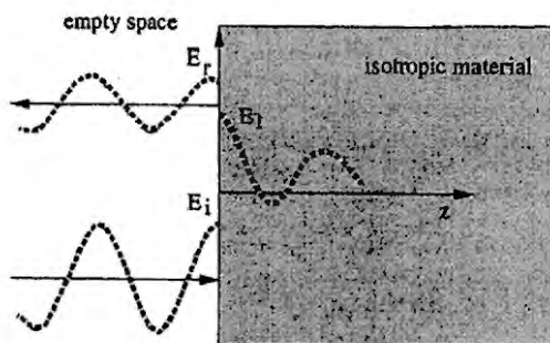
شكل (7.1): الضوء الساقط والمنعكس والنافذ عند سطح المادة ( z=0 ).
