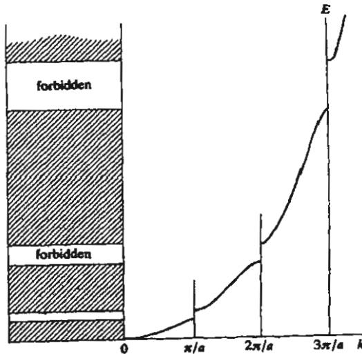
شكل (6.8): شرائط الطاقة وانقطاع E(k) عند حدود مناطق برلوان. لاحظ أن اتساع الشريط يزداد مع زيادة طاقة الشريط.
