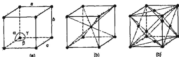
الشكل (1.10): (a) المكعبة البسيطة. (b) المكعبة مع نقطة في مركز المكعب. (c) المكعبة مع نقطة في مركز كل وجه من وجوه المكعب
