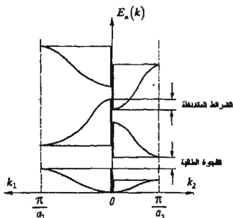
شكل (6.7): E_n(k) باتجاهات مختلفة للمتجه الموجي (k) .
