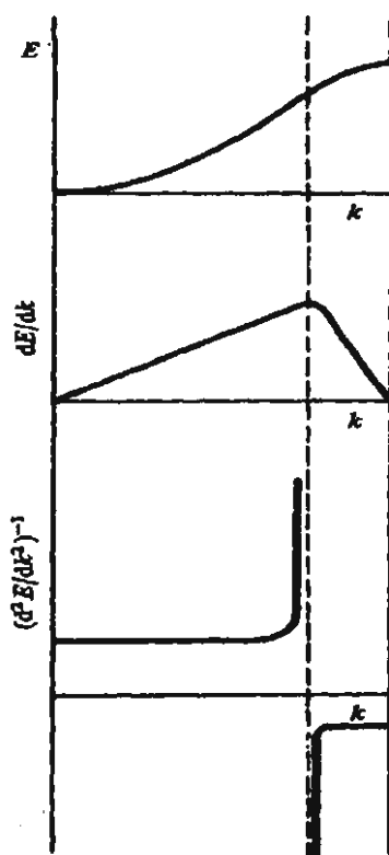
شكل (6.13): السرعة \left(\frac{dE}{dk}\right) والكتلة الفعالة m^* \sim \left(\frac{d^2E}{dk^2}\right)^{-1} ضمن الشريط E(k) في منطقة برلوان الأولى.
