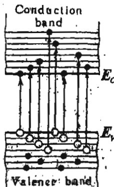
الشكل (6.14): انتقال الإلكترونات من شريط التكافؤ إلى شريط التوصيل عند التسخين. الدوائر السوداء هي الإلكترونات والدوائر البيضاء هي الثقوب.
