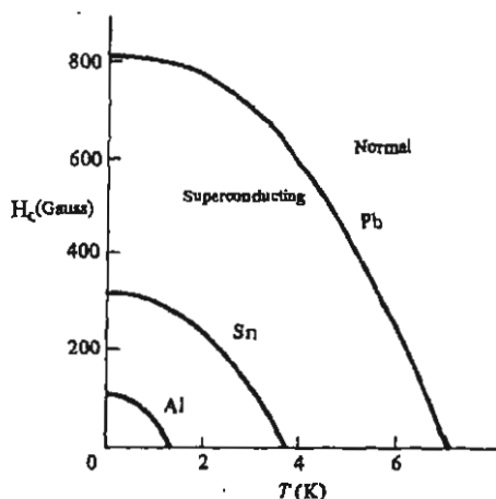
الشكل (9.2): يؤثر المجال المغناطيسي على الحالة فائقة التوصيل بأن يجعل T_c تتراجع إلى قيم أقل.
