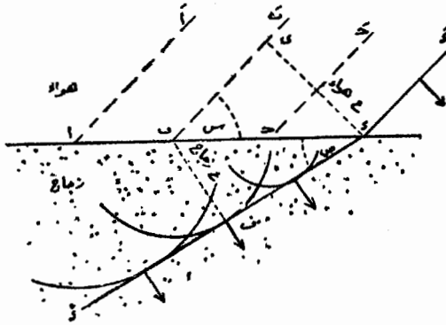
شكل (٣-١٦) تفسير هيجنز لانكسار الضوء
