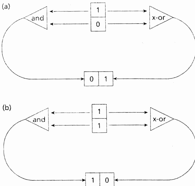
الشكل ١٤-٣ (أ) جهاز الإضافة ينجز 1 = 0 + 1 ، (ب) ينجز 10 = 1 + 1
